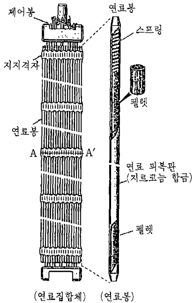
<그림 4> 원자력 연료 모형
