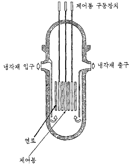
<그림 5> 원자로 모형
