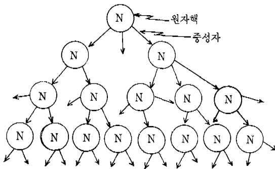
<그림 3> 핵분열 연쇄반응
