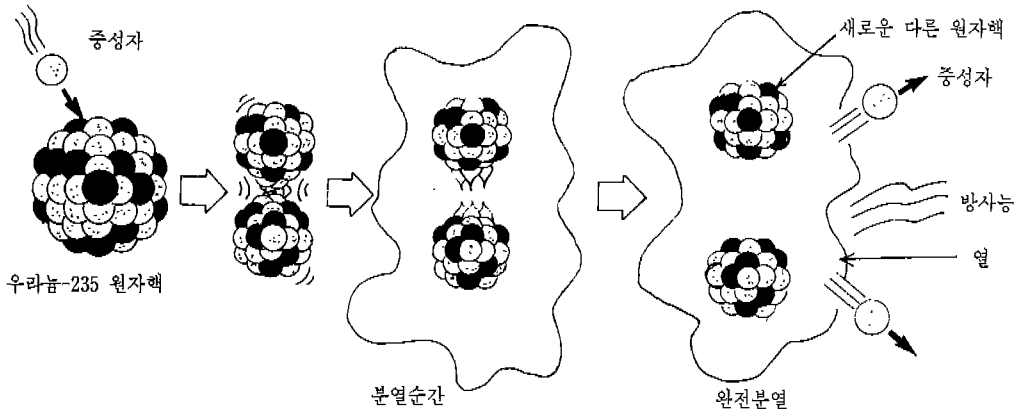
<그림 2> 핵의 분열과정
