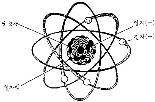
<그림 1> 원자의 구조
