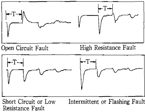
<그림 3> 대표적인 과도시의 전류파형
