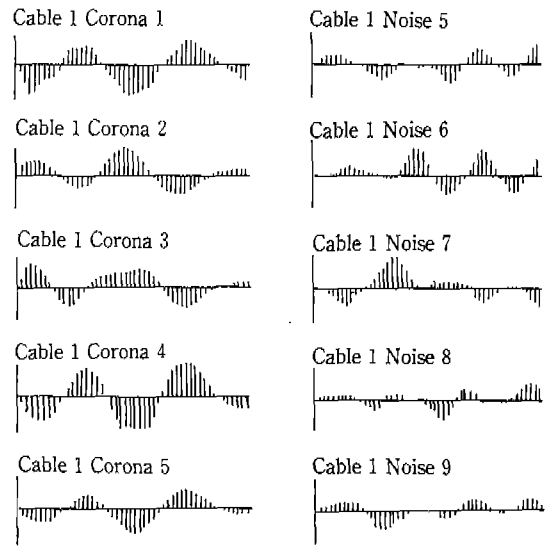
<그림 7> 학습용 입력 Data의 Set
