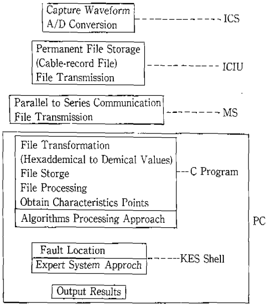
<그림 6> 시스템 구조
