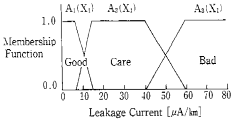
<그림 11> 누설전류 Membership 함수의 구성
