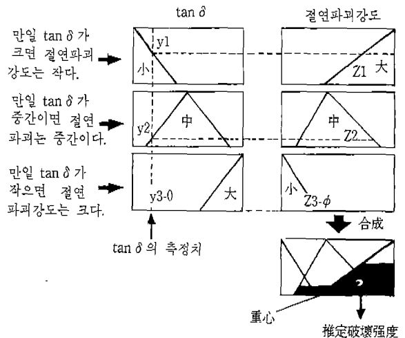
<그림 10> Fuzzy 추론에 의한 절연파괴강도의 추정
