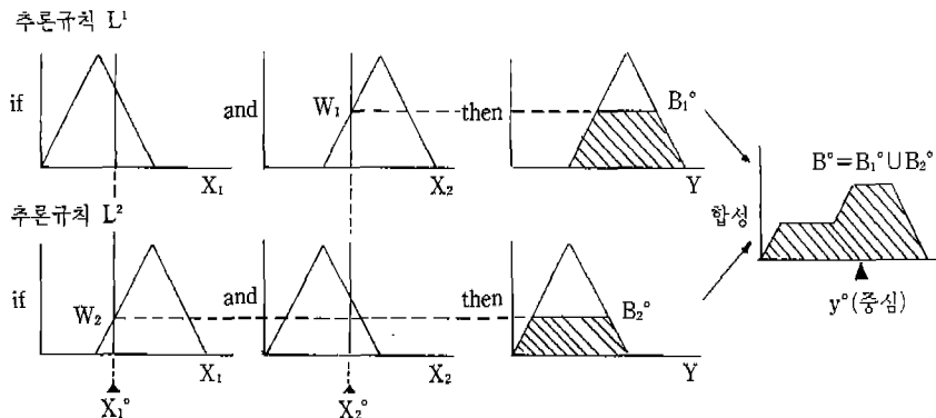
<그림 8> Fuzzy 추론의 개념도
