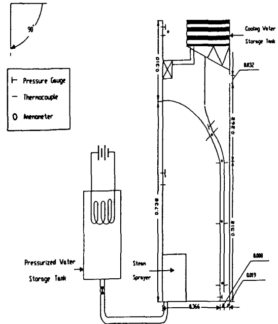
그림2. 서울대의 PCCS 실험장치 개략도
