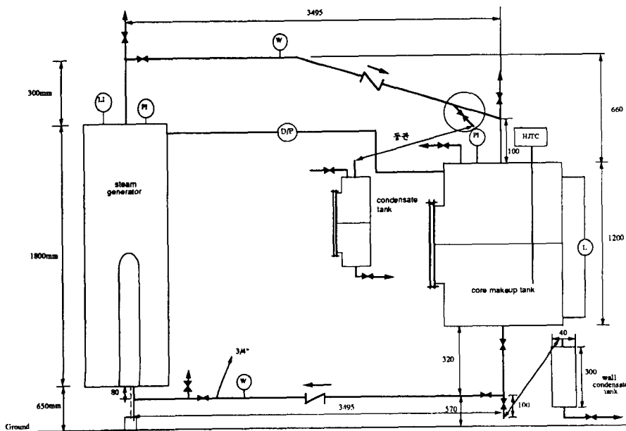
그림 4. 한국과학기술원의 CMT 실험장치 개략도
