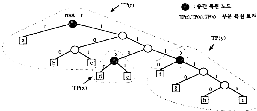
그림 2. 중간 복원 노드와 부분 복원 트리의 예. 여기서 B=(3, 3) 이다. Fig. 2. An example of intermediate decoding nodes and partial decoding trees, where B=(3, 3) .
