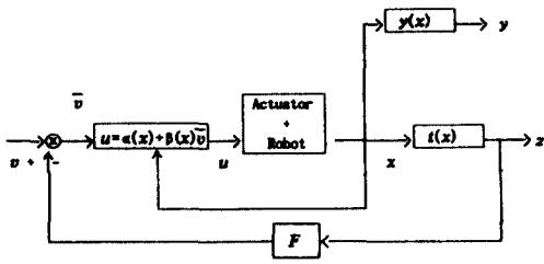
그림 3. 시스템의 안정도를 개선하기 위한 상수이득행렬 (F)을 가해준 시스템도.
