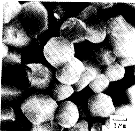
(d) \text{Ca}(\text{Ti}_{0.97}\text{V}_{0.03})\text{O}_3
