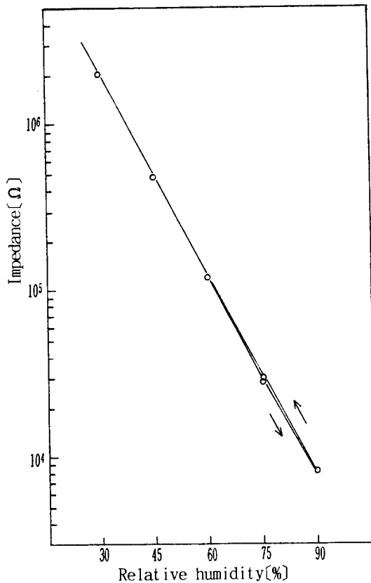
그림 9. 히스테리시스 특성 Fig. 9 Hysteresis characteristics
