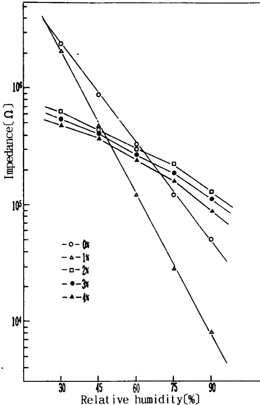
그림 5. 상대습도-임피던스 특성의 V_2O_5 치환량의 의존성
