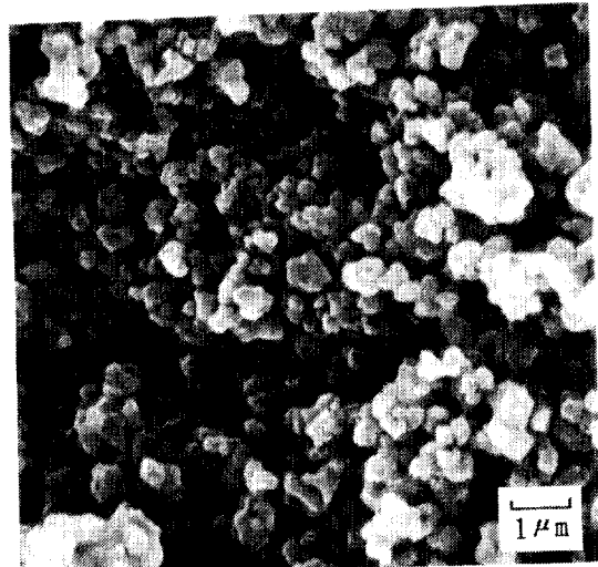
(a) CaTiO_3
