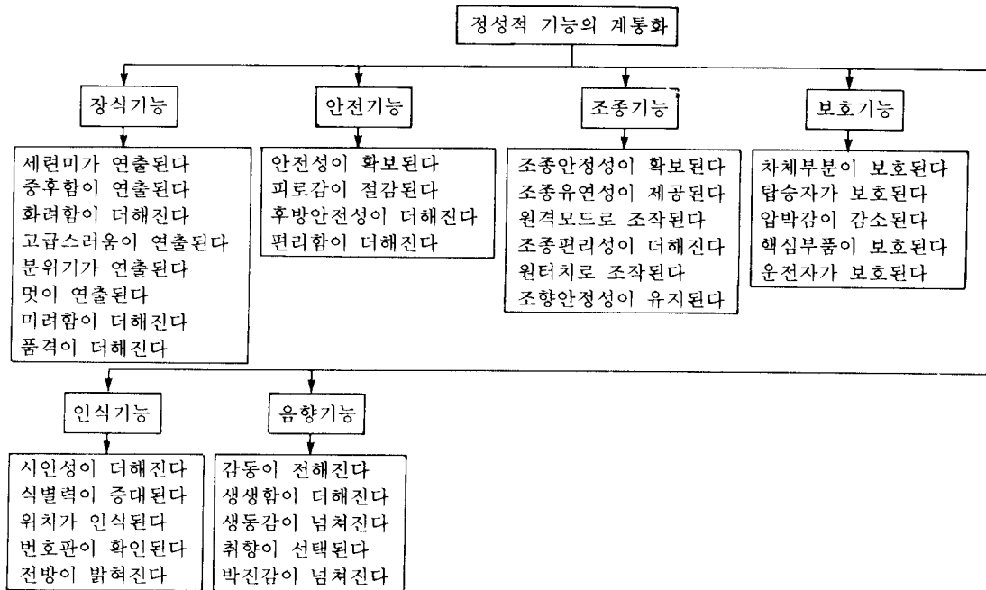
그림 5. 정성적 기능계통도
