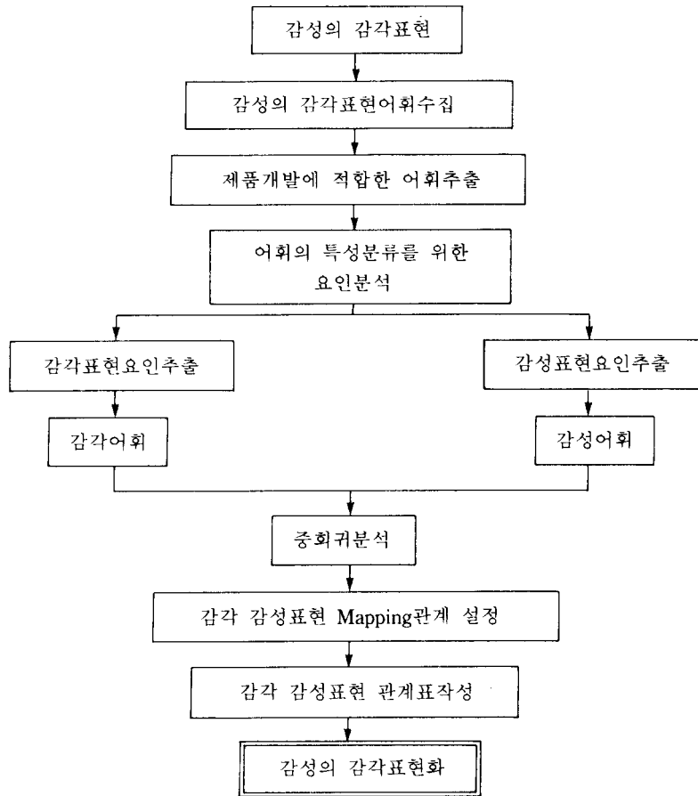
그림 6. 감성의 감각표현화를 위한 흐름도
