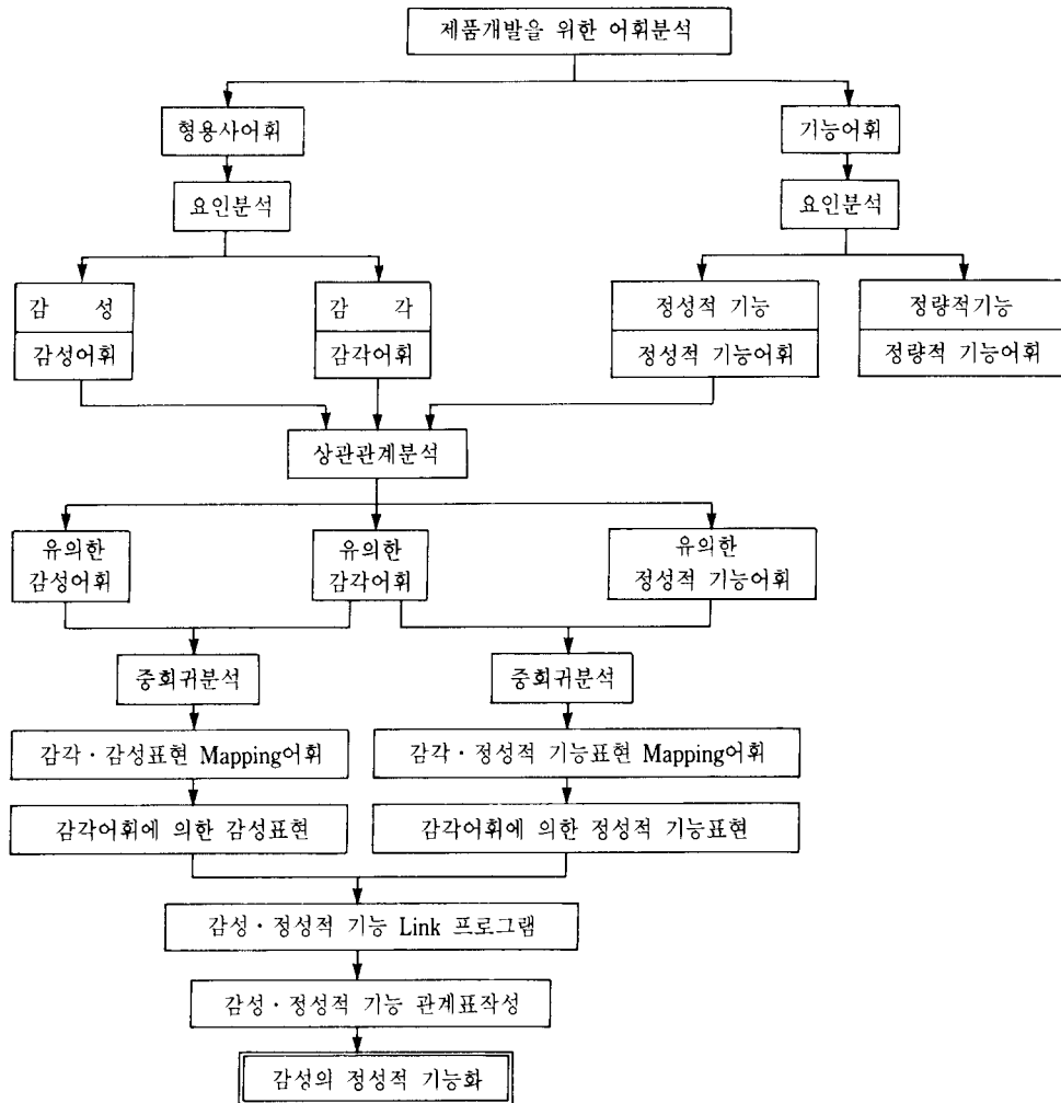
그림 2. 감성의 정성적 기능화를 위한 흐름도
