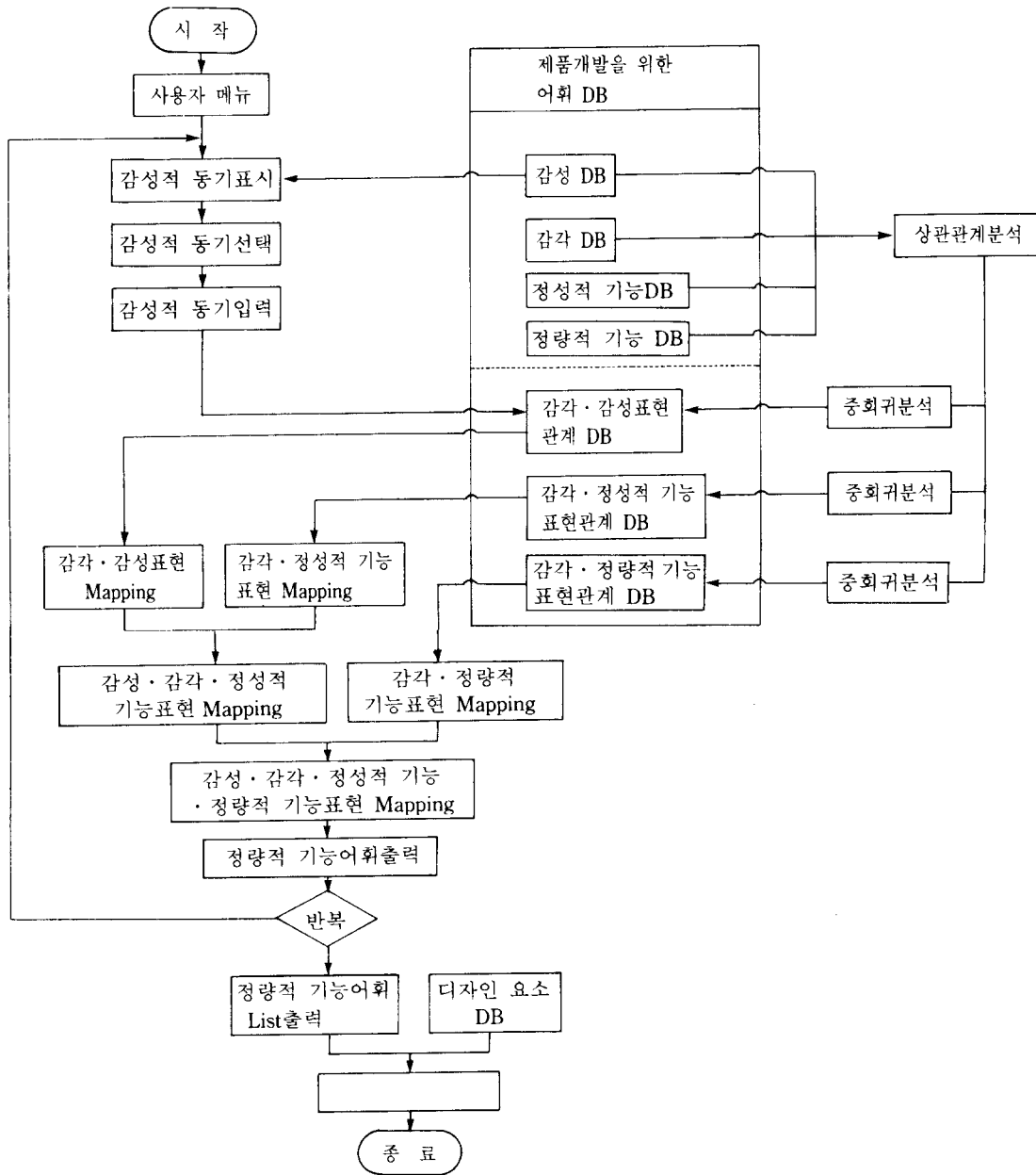
그림 9. 감성적 기능화 시스템구축을 위한 흐름도
