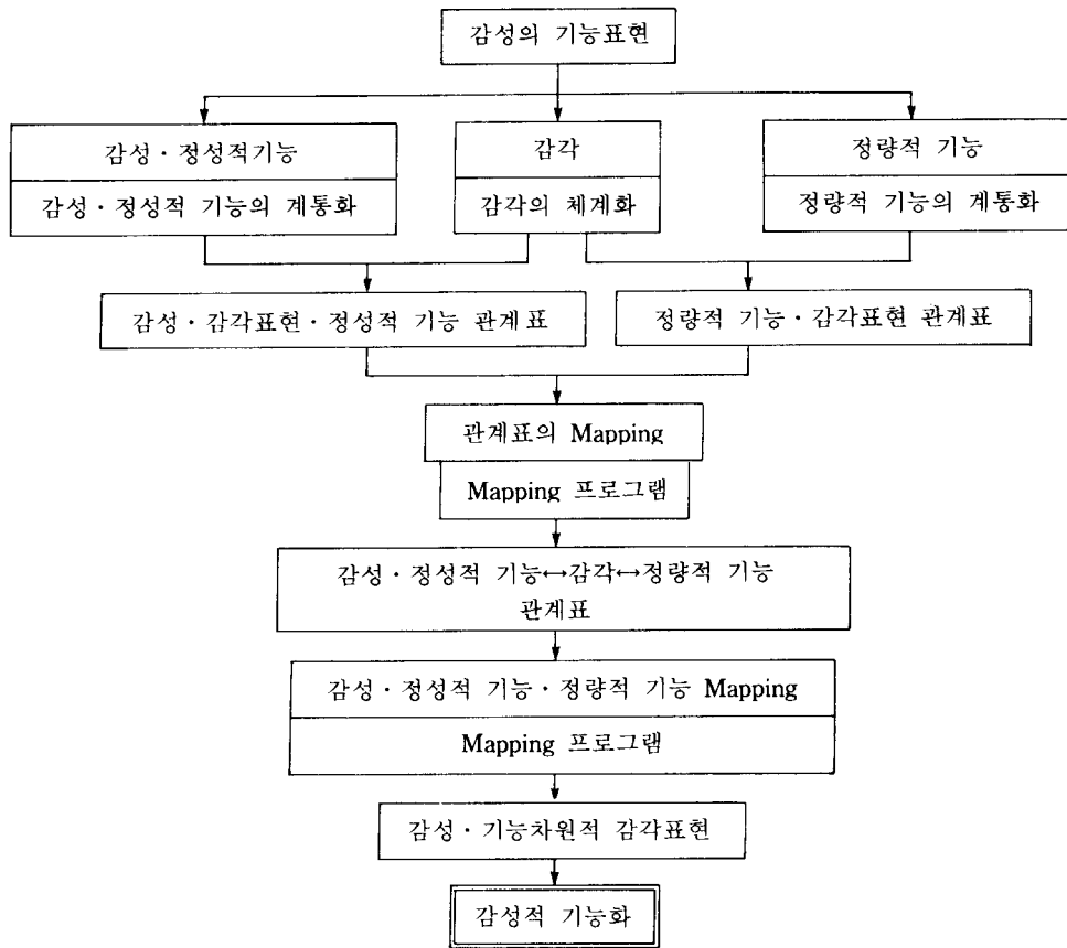
그림 7. 감성적 기능화를 위한 흐름도
