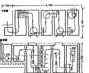
(도 2) 1차처리조의 구조
