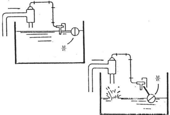
그림2. 후로트 스위치
