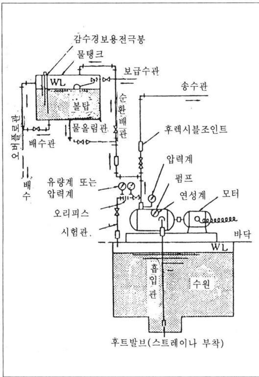
그림1. 수원이 펌프보다 아래에 있는 경우의 물올림장치 등
