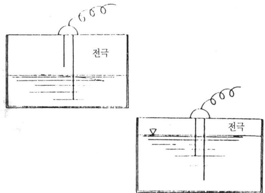
그림3. 전극스위치
