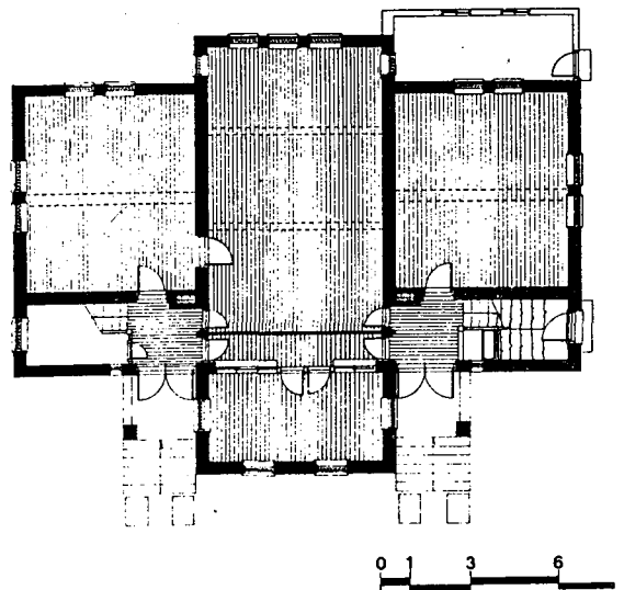
그림3-2 동산성경학교 평면도
