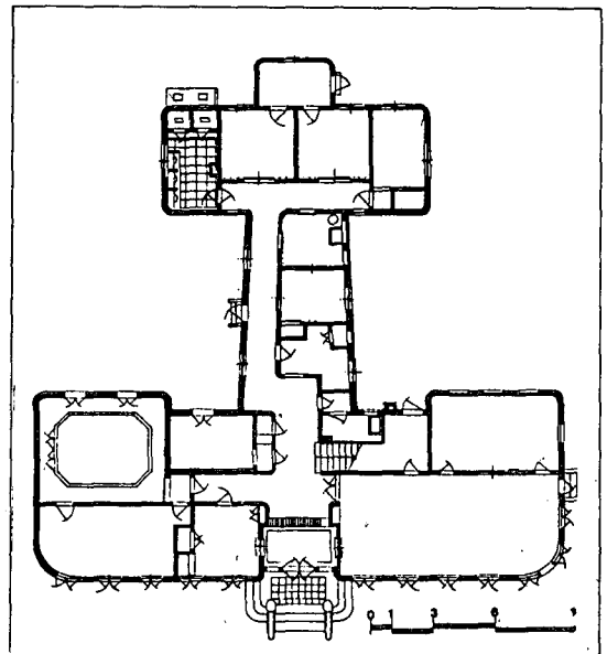
그림3-6 대구측후소 평면도
