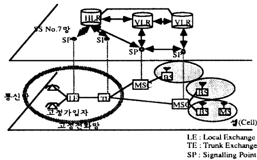
그림 1. 디지털 이동통신 시스템의 구조 Fig. 1. Structure of Digital Mobile Communication System
