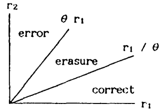
그림. 4 송신 신호가 $S_1(t)$ 일때 수신 신호의 검출영역 Fig. 4 Decision region when $S_1(t)$ was sent
