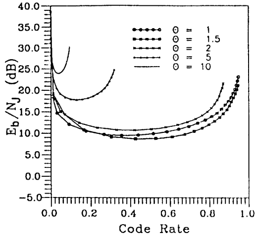
그림. 6 E_c/N_0=10\text{dB} 일때 톤재밍 Fig. 6 Tone jamming at E_c/N_0=10\text{dB}
