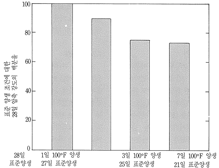
그림 2. 초기 양생 온도가 높을 경우의 강도변화
