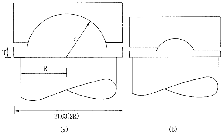
그림 6. 구형좌대 블록
