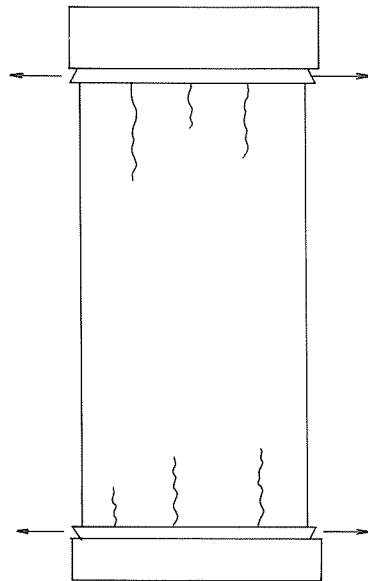
그림 4. 방사응력을 일으키는 연질캐핑재료의 횡방향 흐름
