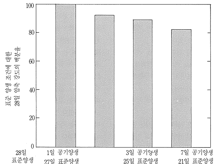
그림 3. 초기 상대습도가 낮은 경우의 강도 변화
