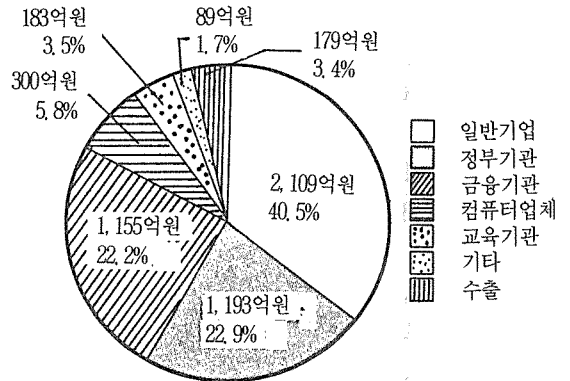
〈거래선별 정보처리매출〉
