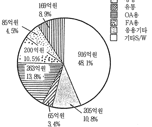
〈S/W종류별 매출액〉
