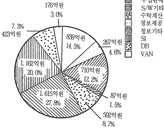
〈S/W종류별 매출액〉
