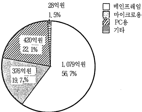
'90년도
