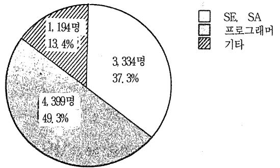
<S/W인력현황>
