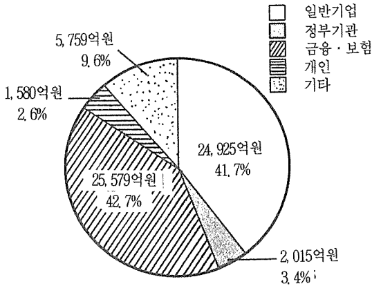
<정보통신부문 거래선>
