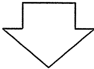
'90년도
