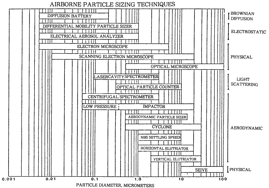
그림 2. 에어로졸 측정기기들의 측정 범위
