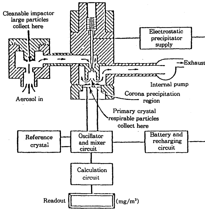
그림 10. 호흡성 입자 포집용 압전식 미세질량기(Piezoelectric Microbalance)의 구조도
