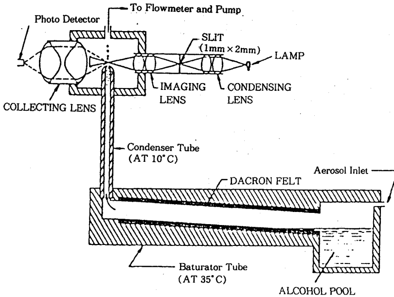
그림 9. 연속유동 응축핵 계수기(Condensation Nucleus Counter)의 구조도
