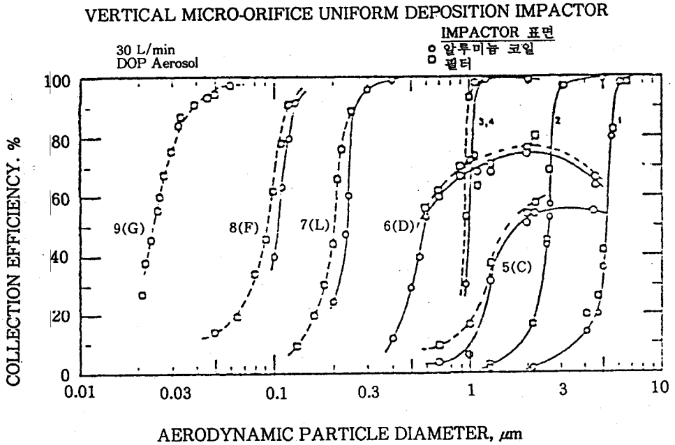
그림 7. 다단식 마이크로 오리피스 충돌기(Micro-Orifice Impactor)의 입자분리 성능곡선
