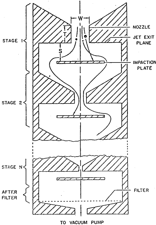
그림 6. 다단 계단식 충돌기(Multi-stage Cascade Impactor)의 구조도
