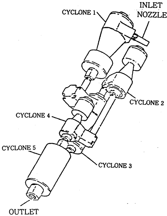
그림 8. 5단 계단식 사이클론 분리기 (Cascade Cyclone Separator)의 구조도
