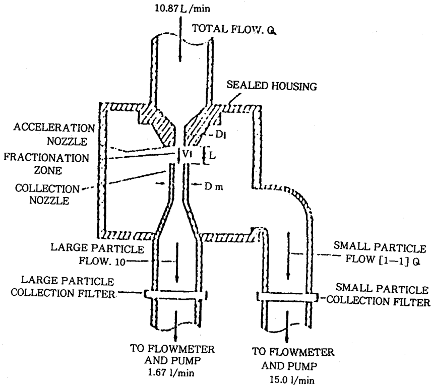
그림 4. 이분법 샘플러의 구조 개략도(Dichotomus Sampler)
