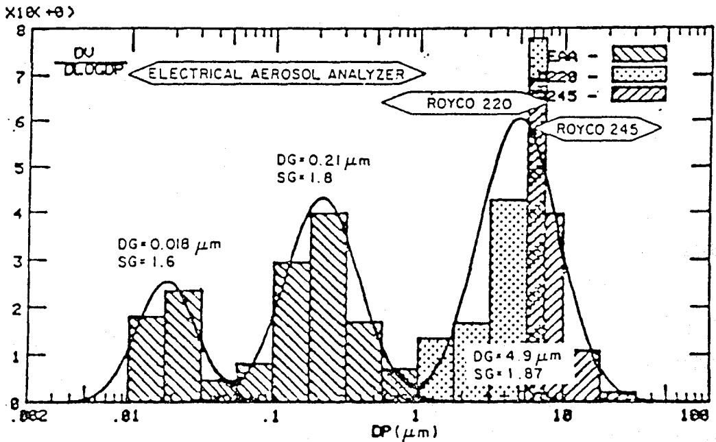
그림 1. 대기 에어로졸의 trimodal 크기 분포
