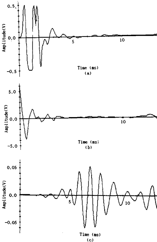
그림 2 (a) 1kHz 자극음이 포함된 유발이음향 신호, (b) 유발이음향 방사신호를 자기상관법으로 처리한 신호, (c) 유발이음향 방사신호를 상호상관법으로 처리한 신호
