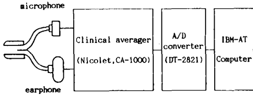
그림 1 유발이음향방사 측정 및 처리 시스템
