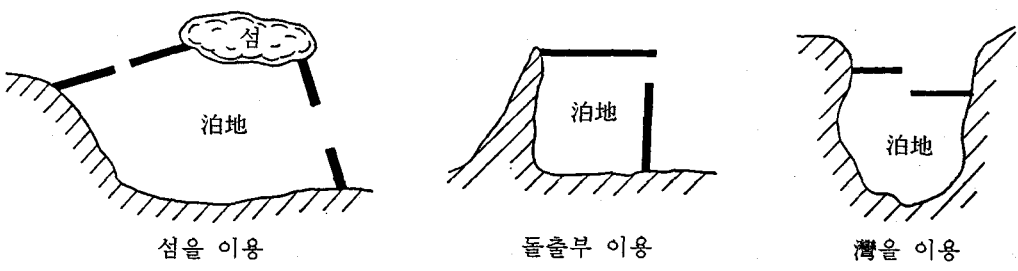
자연의 지형을 이용한 방파제 배치 예
