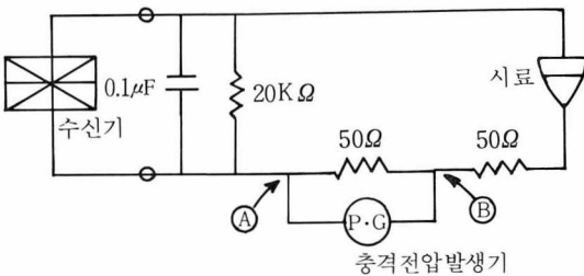
<그림 1> 시험회로
