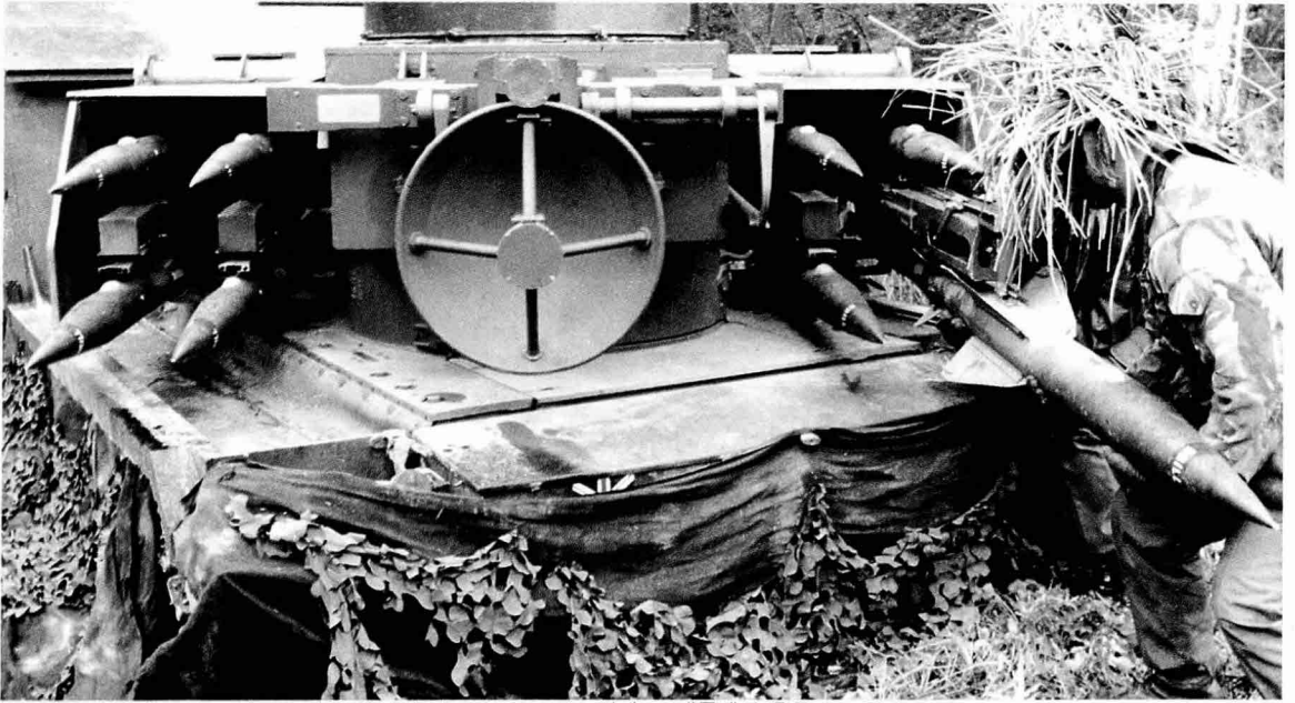
▲ 영국 궤도형 Rapier 저고도 방공 미사일 시스템. Rapier는 현재 13개국에서 운용되고 있다
