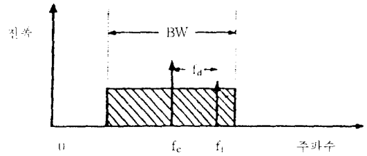
그림 1. 톤 간섭파의 스펙트럼 Spectrum of tone interferer.
