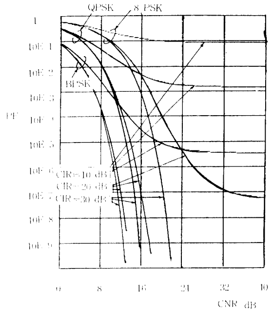
그림 13. 다중 간섭과 가우시안잡음에서의 PSK 신호의 오류율 Error rate of PSK signal influenced by multiple interferer and Gaussian noise.
