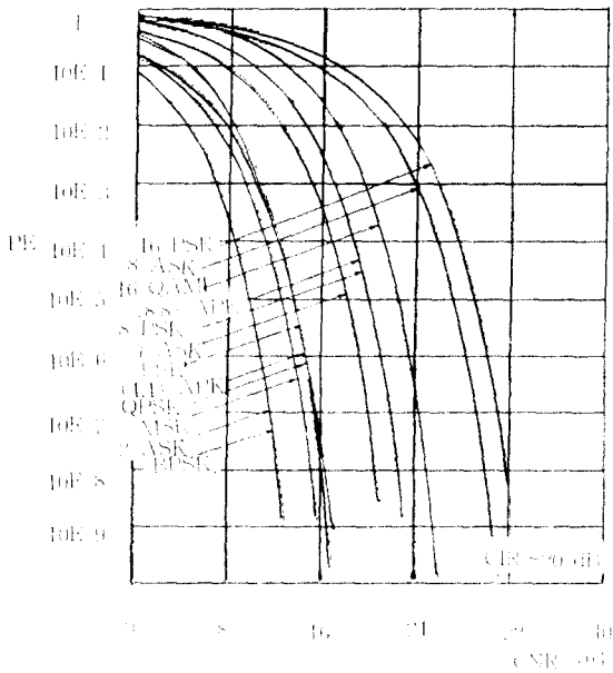
그림 22. 단일 음파에 의한 간섭과 가우시안 잡음에 의한 다양한 디지털 변조 신호의 오류율 비교 Error rate comparison of various digitally modulated signal influenced by tone interferer and Gaussian noise
