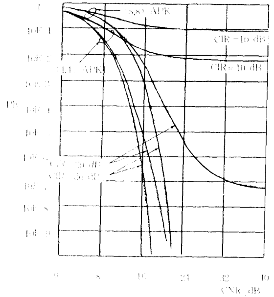
그림 21. 다중 음파에 의한 간섭과 가우시안 잡음에 의한 APK 신호의 오류율 Error rate of APK signal influenced by multiple interferer and Gaussian noise
