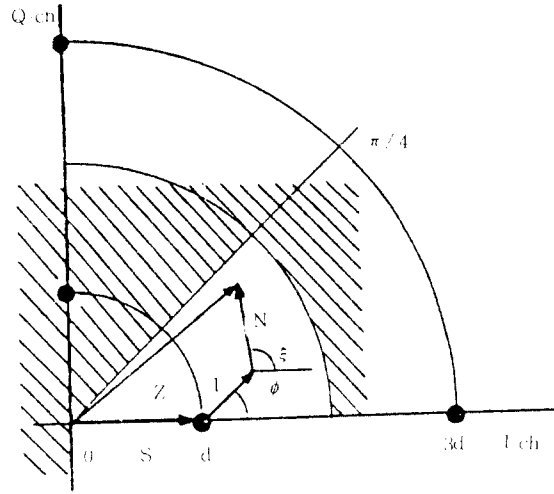
그림 9. 간섭영향하의 APK신호의 수신 케이지도. Phasor diagram of received APK signal with interferer and noise.
