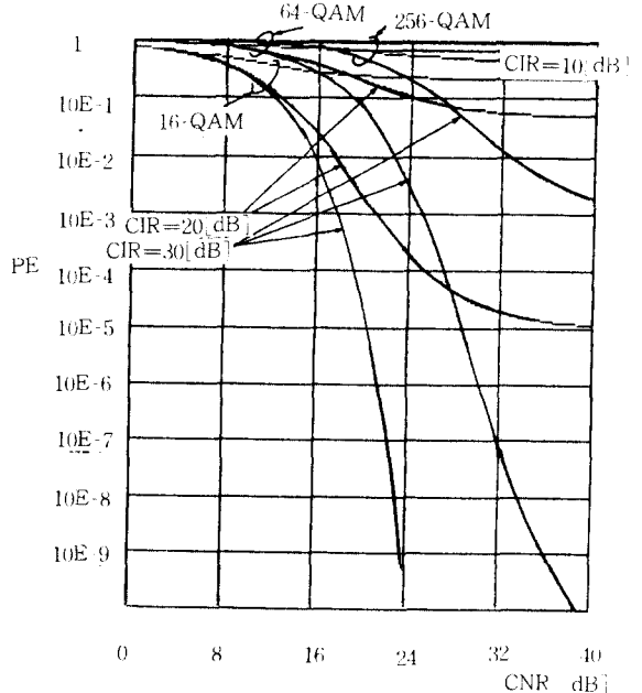
그림 19. 다중간섭과 가우스잡음하의 QAM 신호의 오류 Error rate of QAM signal influenced by multiple interferer and Gaussian noise.
