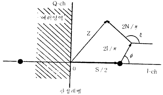
그림 7. 간섭영향하의 MSK 신호의 수신 케이지도 Phasor diagram of received MSK signal with interferer and noise.
