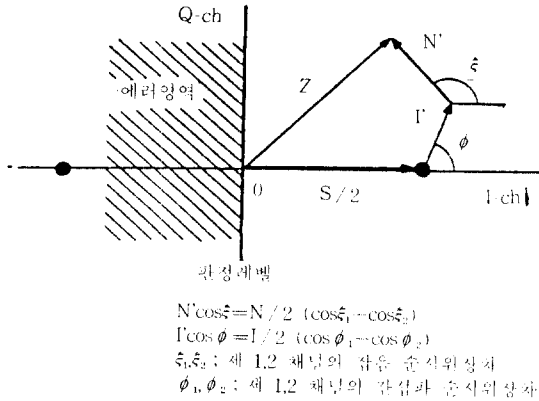
그림 6. 간섭영향하의 FSK 신호의 수신 케이지도 Phasor diagram of received FSK signal with interferer and noise.
