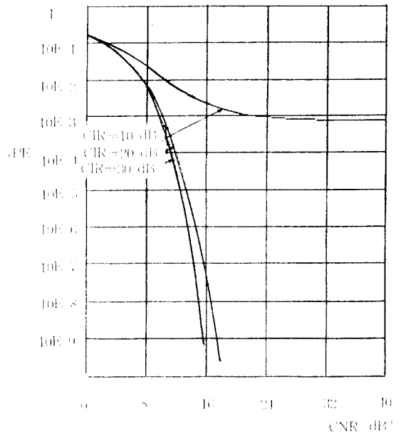
그림 15. 다중 간섭과 가우시안잡음에서의 FSK 신호의 오류율 Error rate of FSK signal influenced by multiple interferer and Gaussian noise.
