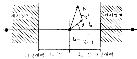
그림 8. 간섭영향하의 QAM신호의 수신 케이지도 Phasor diagram of received QAM signal with interferer and noise.
