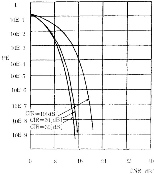
그림 16. 톤간섭과 가우스잡음하의 MSK 신호의 오류 Error rate of MSK signal influenced by tone interferer and Gaussian noise.
