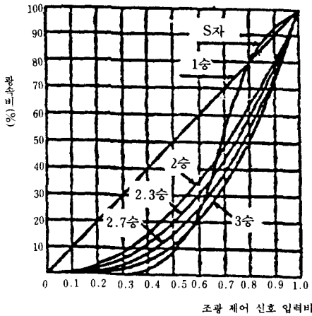
그림 5. 각종 조광 특성 곡선
