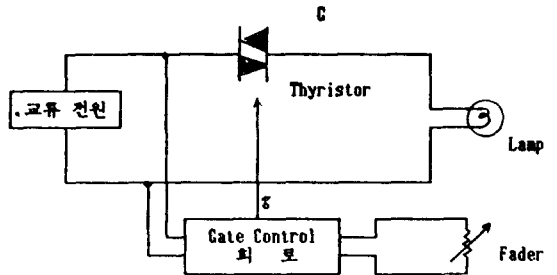
그림 3. Thyristor 조광기의 구성도
