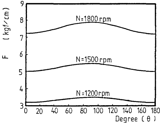
Fig. 4. 캠링에 작용하는 Vane의 慣性力
