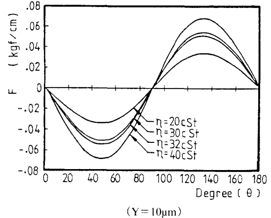
Fig. 5. Vane에 작용하는 粘性力
