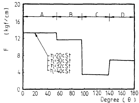
Fig. 9. 垂直方向으로 作用하는 Vane의 合力
