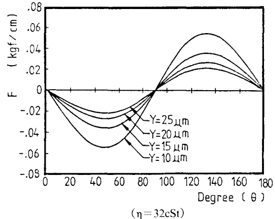
Fig. 6. Vane에 작용하는 粘性力
