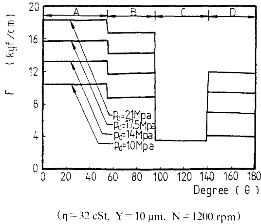
Fig. 11. 垂直方向으로 작용하는 Vane의 합력
