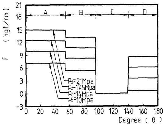
Fig. 7. 壓力에 의한 垂直作用力
