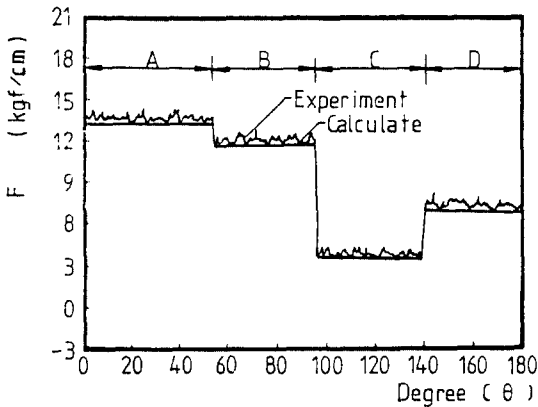
Fig. 8. 垂直方向으로 作用하는 Vane의 合力
