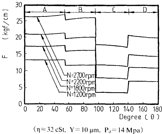
Fig. 12. 垂直方向으로 작용하는 Vane의 합력
