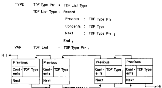
그림 3 데이터 구조 Fig. 3 Data structure
