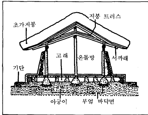
[그림 3] 한옥의 기본구조
