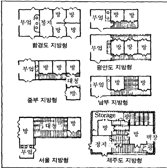
[그림 5] 조선시대 서민주택의 기본 평면형
