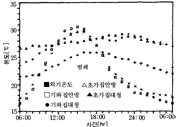
[그림 8] 하계 자연실온 변화
