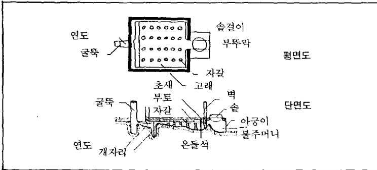
[그림 6] 재래식온돌의 구조
