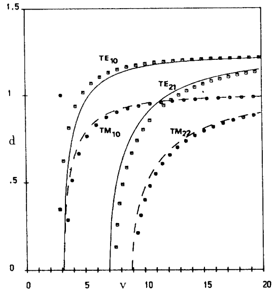
그림4. \epsilon_s=1.0, \epsilon_o=1.5 일때 유전체 구형도파관의 분산특성 Dispersion characteristics for dielectric waveguide with relative permittivity, \epsilon_s=1.0, \epsilon_o=1.5 , respectively
