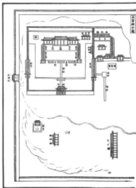
그림-4. 肅宗代의 永寧殿圖(『宗廟儀軌』에서)
