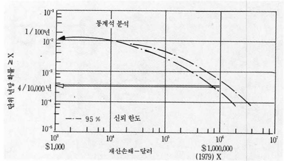
그림2. Exxon사의 위험 손실 정보 시스템에 따른 HPI 설비에서 1961~1975에 발생한 화재 / 폭발
