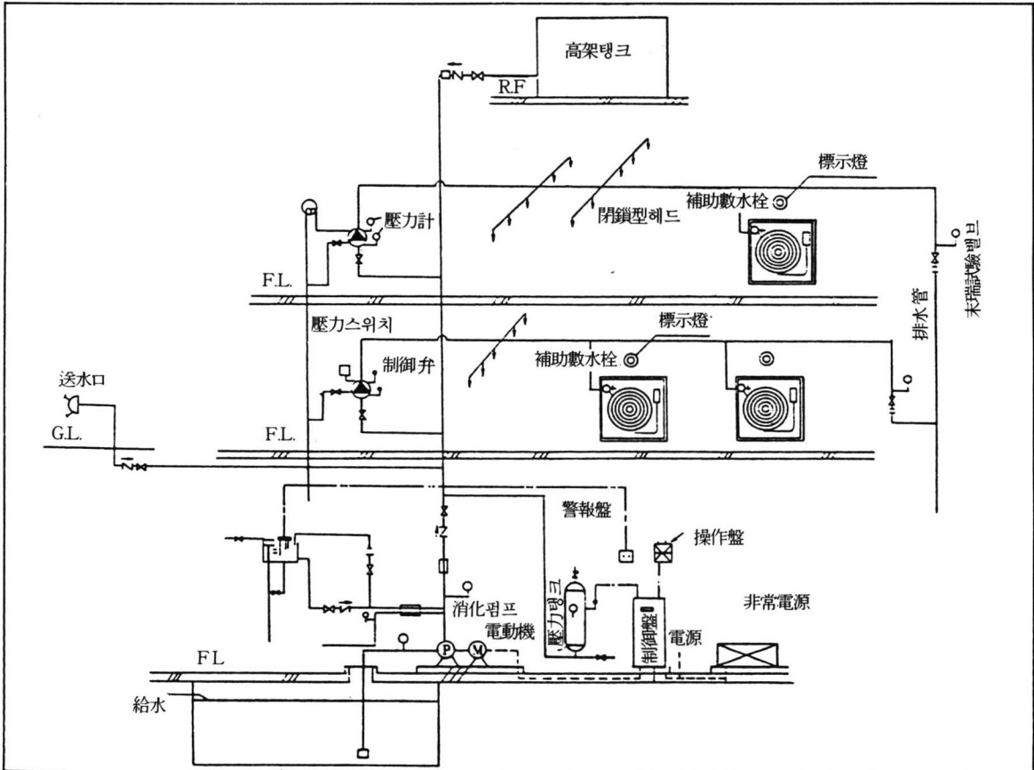
(그림1) 보조소화전을 설치한 Sprinkler
