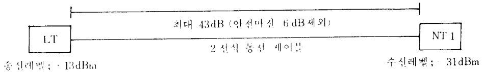
그림 7 U-트랜시버의 최소 수신레벨 Level diagram of U-tranceiver system.
