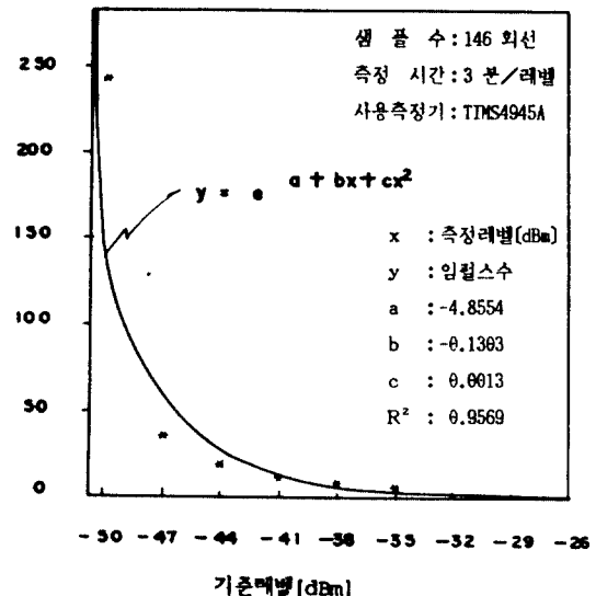
그림 6 평균 임펄스 발생수(9) Average number of impulse.
