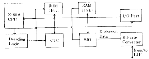
그림 3 Control part의 구성도 Block diagram of control part.
