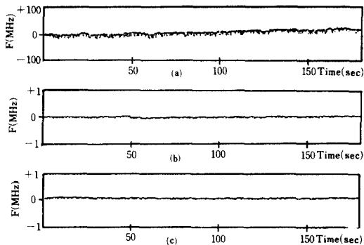
그림 7 주파수 드리프트 특성곡선 (a) 자유동작시 (b) 주파수 안정시 (c) 주파수-출력안정시 Frequency drifts of (a) free running (b) frequency stabilized (c) frequency-output power stabilized state.
