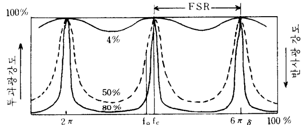
그림 2 반사율에 따른 F-P 간섭계의 출력특성 F-P interferometer characteristic of output power to reflectivity.
