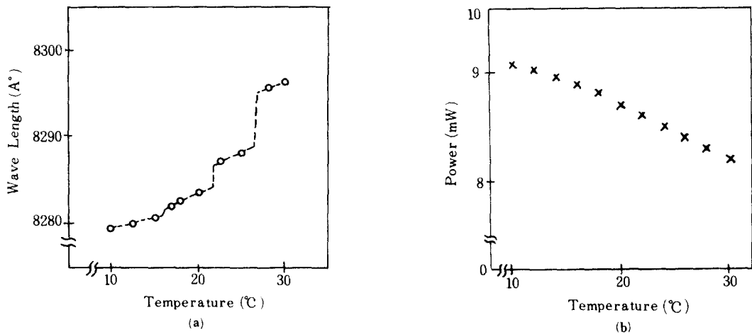
그림 4 반도체 레이저의 주파수-온도, 출력-온도특성곡선 (a) 주파수-온도특성 (b) 출력-온도특성 Experimental results of frequency and output power versus temperature. (a) Frequency-temperature (b) Output power-temperature.
