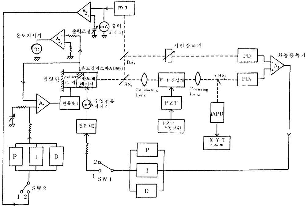
그림 1 F-P간섭계를 사용한 반도체 레이저 주파수-출력 인 정화 시스템 실험장치 Experimental setup for measurement the charac- teristic of both frfrequency and output power stabilized semiconductor laser using F-P interfe- rometer.
