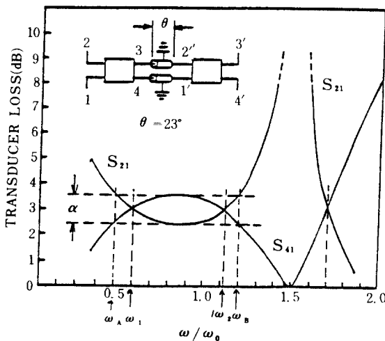
그림 2 강한 磁氣結合을 가지는 2단 90° 하이브리드에 대한 應答特性的 計算值 Computer-Generated Characteristics of Two-Stage Quadrature Hybrid with Tight Magnetic Coupling.
