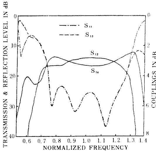
그림 8 集中定數型 廣帶域 90° 하이브리드의 周波數特性 Frequency Characteristics for the Broadband Lumped-Element 90° Hybrid ( C_1=78.67 , C_2=67.80 , C_{s1}=89.08 , C_{s2}=44.54 , C_M=25.93 \mu F , L_{s1}=0.02693 , L_{a1}=0.1139 , L_{a2}=0.04866 , L_s=0.05667 , L'_s=0.0 , L_M=0.04121 \mu H ).
