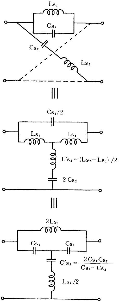
그림 A4 第2次 遲延等化器 Secon-Order Delay Equalizer.
