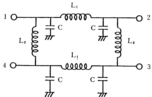
그림 3 (a) 磁氣結合을 갖지 않는 基本的인 集中定數型 90° 하이브리드 Fundamental Lumped-Element 90° Hybrid without Magnetic Couplings ( L_1 = Z_0 / \sqrt{2} \omega_0 , L_2 = Z_0 / \omega_0 , C = (1 + \sqrt{2}) / \omega_0 Z_0 )
