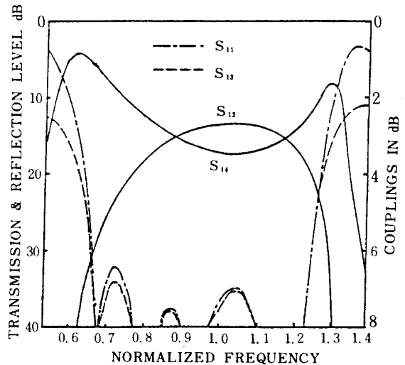
그림 6 (b) 7단 브랜치가이드 하이브리드의 應答特性 Response Curves for 7-Branch-Guide Coupler ( C_1=19.88 , C_2=55.77 , C_3=107.5 , C_4=145.24 pF, L_{a1}=1.255 , L_{a2}=0.3352 , L_{a3}=0.07945 , L_{a4}=\infty , L_{b1}=0.02102 , L_{b2}=0.04993 , L_{b3}=0.0357 , L_{b4}=0.0219 \mu H).
