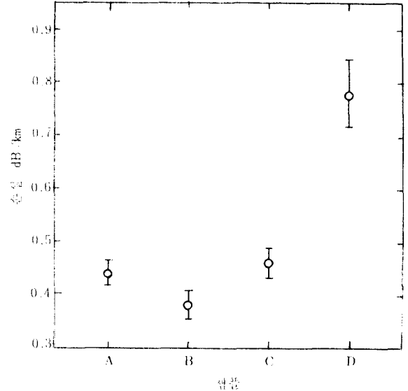
그림 9 단일모드 광섬유의 손실 측정 결과 Result of Loss Measurement of Single Mode Optical Fibers.
