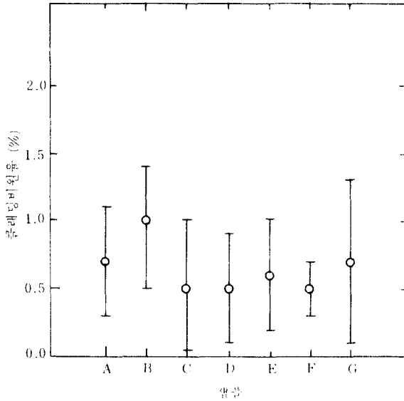
그림 7 다중모드 광섬유의 클래딩 비원율 측정 결과 Result of Cladding Non-Circularity Measurement of Multimode Optical Fibers.
