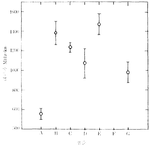
그림 2 다중모드 광섬유의 대역폭 측정 결과 Result of Bandwidth Measurement of Multi-mode Optical Fibers.
