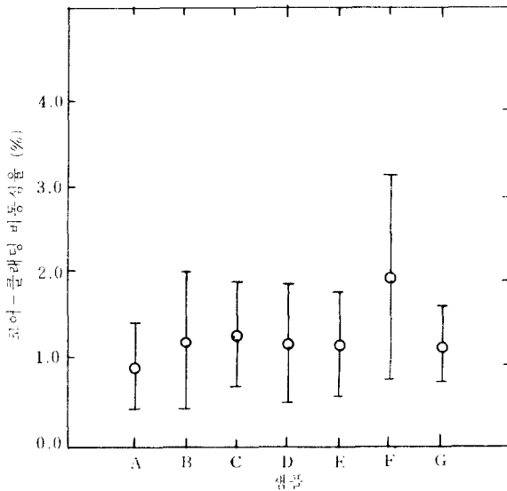
그림 8 다중모드 광섬유의 코어-클래딩 비동심율 측정 결과 Result of core-cladding non-concentricity Measurement of multimode optical fibers.
