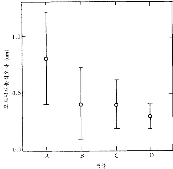
그림12 단일모드 광섬유의 모드 필드 동심오차 측정 결과 Result of mode field concentricity error measurement of single mode optical fibers.
