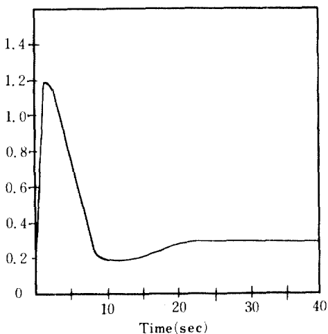
그림 5 온도 20°C에서 19°C로 변환시의 과도응답 특성 Transient response of the temperature change from 20°C to 19°C.
