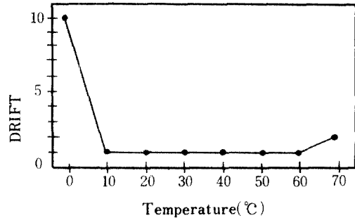
그림 7 설정 온도에 따른 온도 변화 특성 Characteristic of temperature drift for 10 minutes at each set point.
