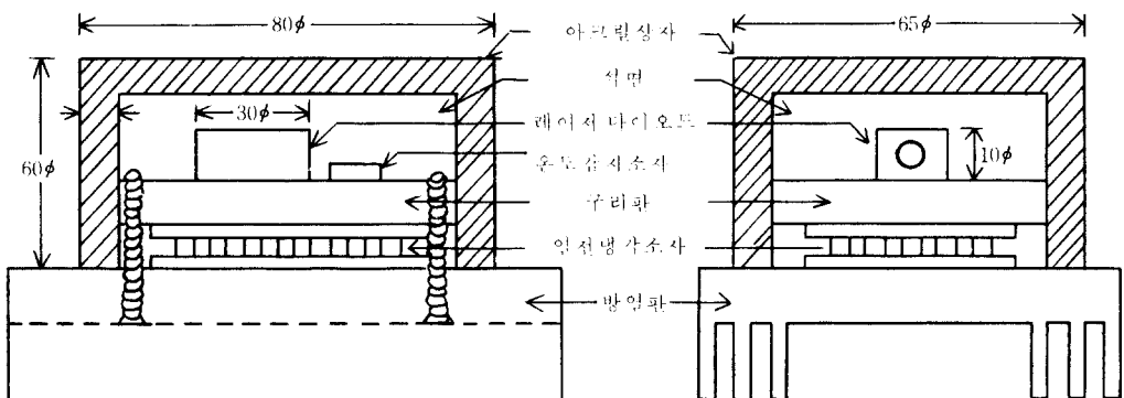
그림 3 恒溫器의 幾何學的 構造 Construction of thermal chamber.
