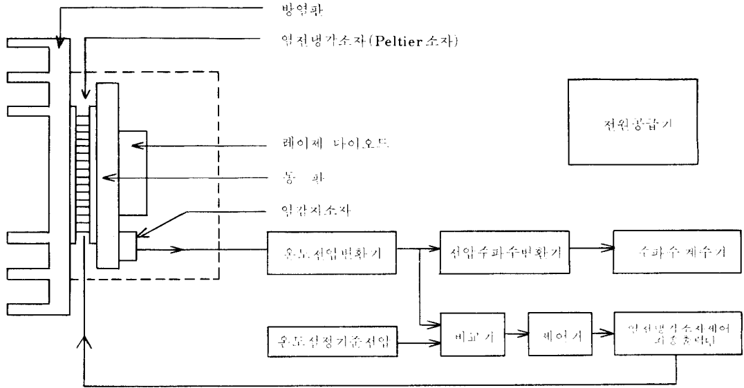
그림 2 온도 조절 및 측정 시스템의 기본 계통도. Fundamental diagram for temperature measurement and control system.
