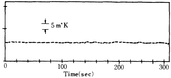
그림 6 설정 온도 20°C에서의 시간에 따른 온도변화 특성 Temperature drift at 20°C for 5 minutes.
