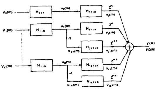
그림 9 多相回路(그림8)의 等價回路 Equivalent system of the polyphase network.
