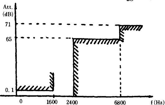
그림 4 原型式필터의 減衰特性 Attenuation of prototype filter.
