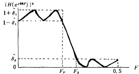
그림 5 原試型필터의 特性
