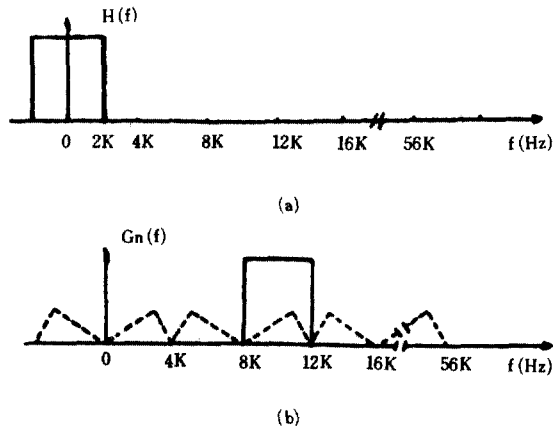
그림 2 原試型필터와 채널필터의 特性 (a) 理想的인 原試型필터의 特性 (b) 채널2의 信號를 추출하는 채널필터의 特性
