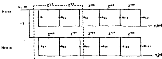
그림 10 곱셈회수를 줄이기 위한 필터의 構造 FIR filter structure for the reduction of multiplication rate.
