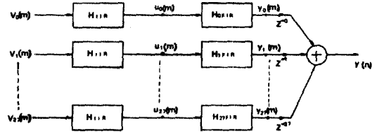
그림 8 多相回路의 IIR部分과 FIR部分 IIR and FIR part of polyphase network.
