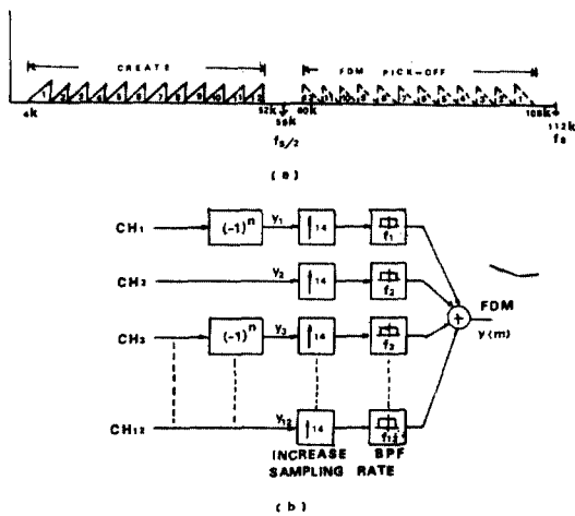
그림 1 BPF로 이루어지는 TDM/FDM變換器 (a) 12채널 TDM/FDM變換器의 周波數分布
