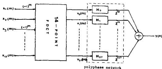
그림 3 多相回路与 FDCT로 이루어지는 TDM/FDM變換器의 構成 TDM/FDM translation with the polyphase network and fast DCT.
