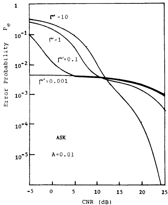
그림 7 \Gamma' 의 변화에 따른 ASK 신호의 오류 The error probability of ASK signal with impulsive index \Gamma' .
