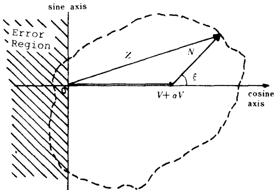
그림 2 수신 FSK 신호의 합성 페이저도 ( a_k=1 ) The phasor diagram of received FSK signal ( a_k=1 ).
