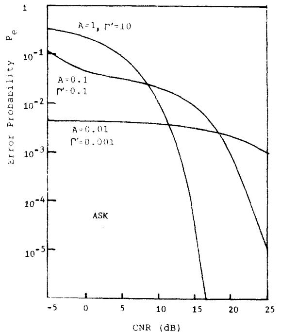
그림 5 임펄스 지수에 의한 ASK 신호의 오류 The error probability of ASK signal with impulsive index.
