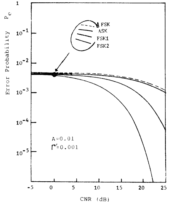
그림 9 임펄스성 잡음 환경하에서 AFSK 신호의 오류 The error probability of AFSK signal in the environment of impulsive noise.
