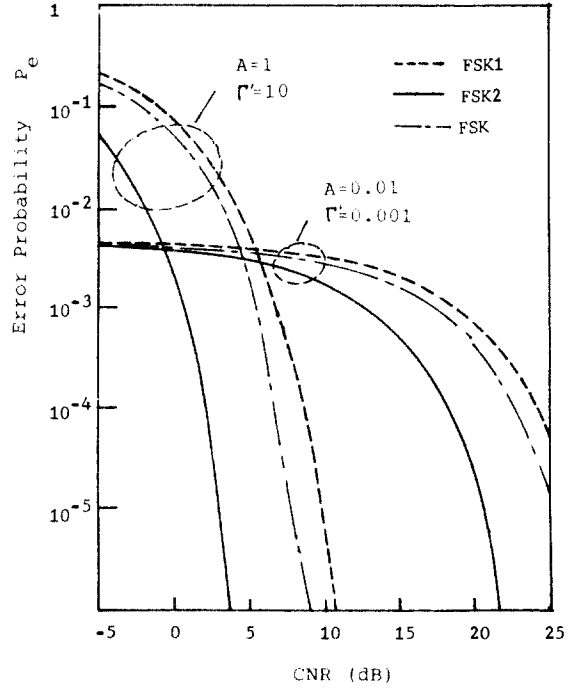
그림 8 임펄스노이즈에 따른 FSK 신호의 오류 The error probability of FSK signal with impulsive index.
