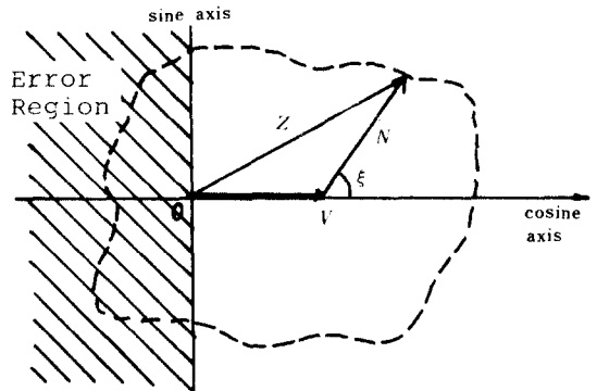
그림 3 수신 FSK 신호의 합성 페이저도 ( a_k=0 ) The phasor diagram of received FSK signal ( a_k=0 ).
