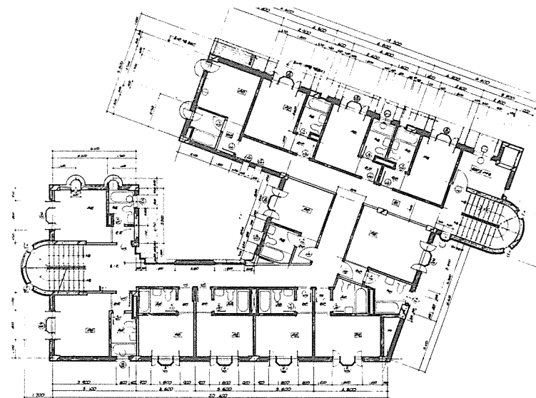
3 층 평면도
