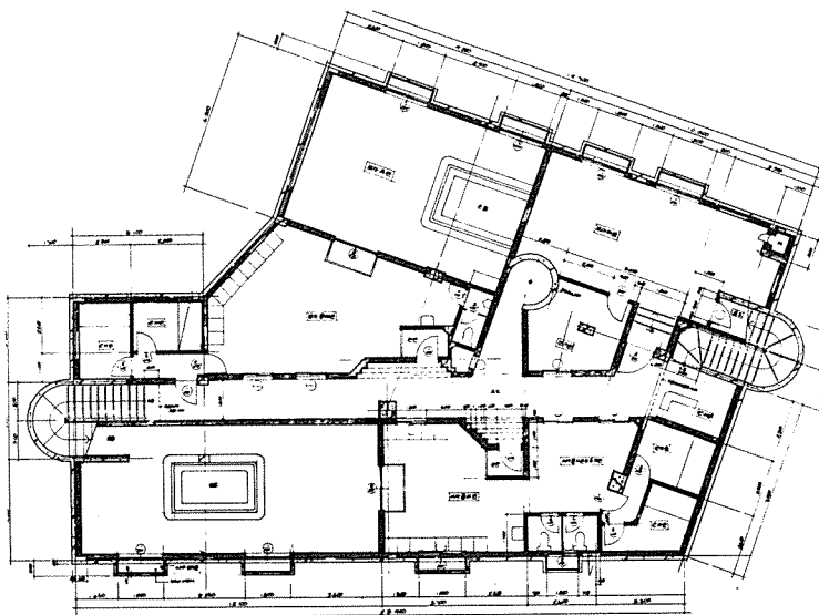
지하층 평면도
