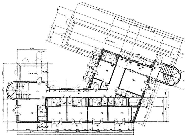
4 층 평면도
