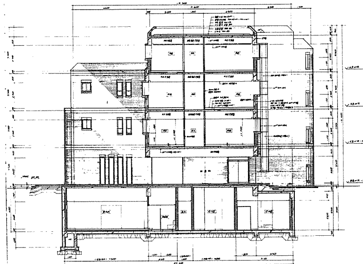
단면도
