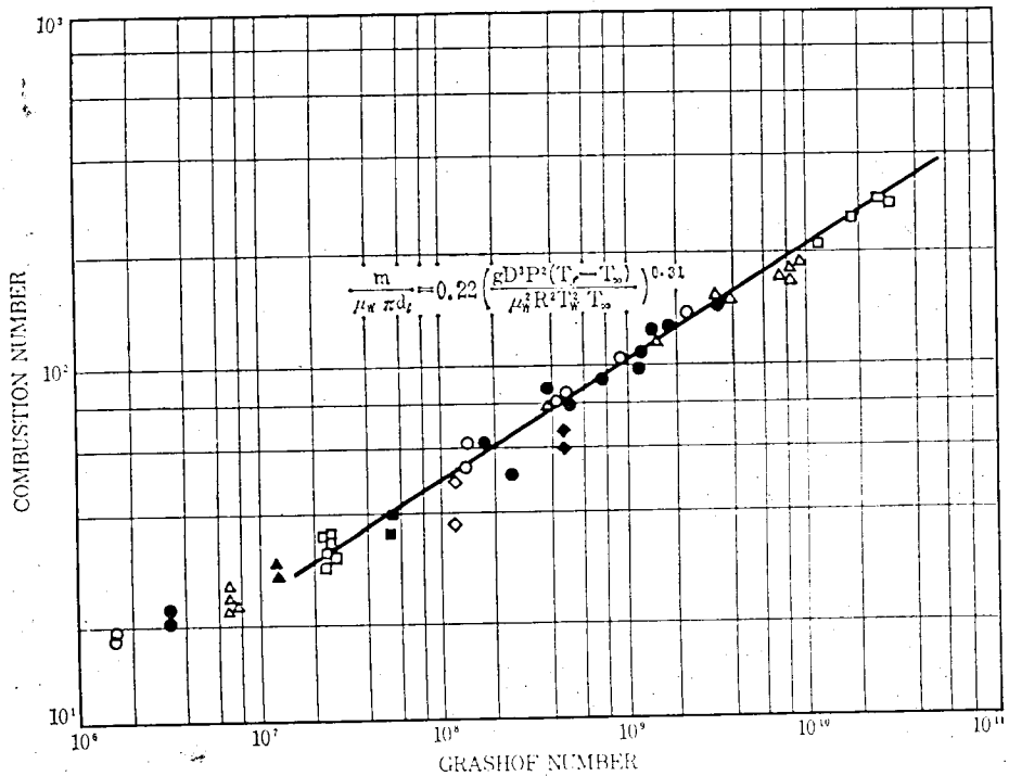
〈그림 5〉 Plexiglas tube의 内部燃焼速度와 Grashof數의 關係 Combustion Number = m / \mu_w \pi d ( \propto 燃焼速度) Grashof Number = \frac{g D^3 \rho^2 (T_f - T_w)}{\mu_w^2 R^2 T_w^2 T_\infty} , W = \text{wall} .
