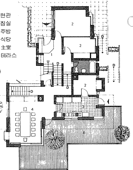
평면도
