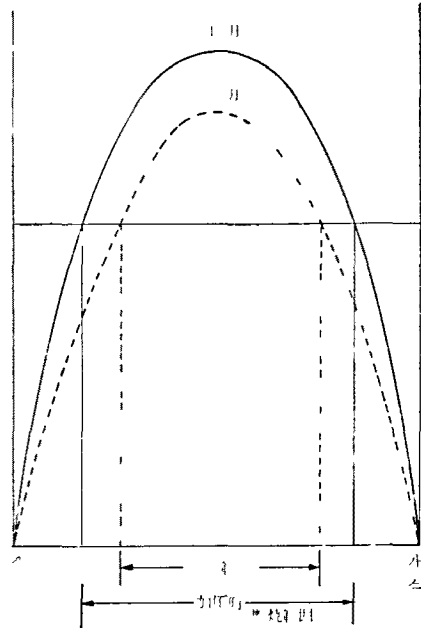
(그림 2) 高壓에 의한 燃焼範圍
