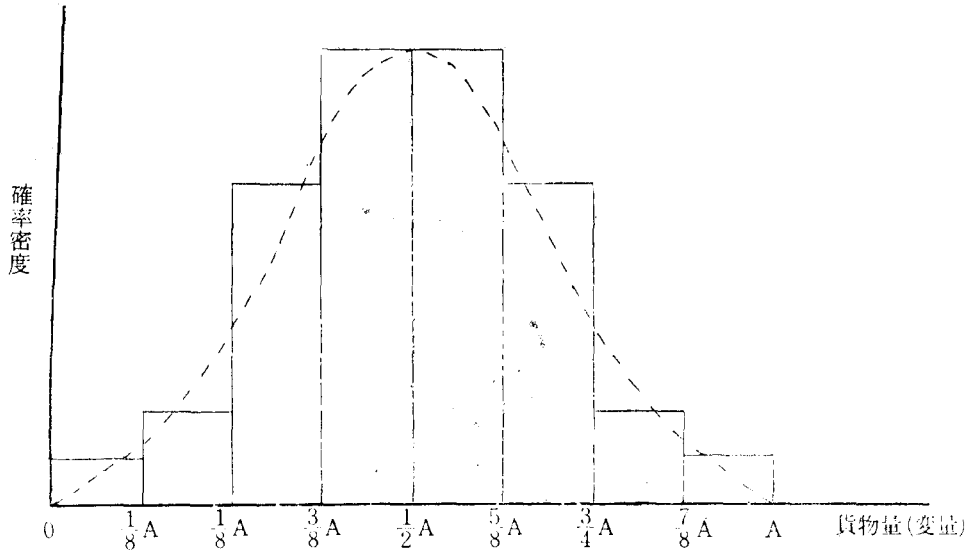
(그림 2) 航海當 貨物의 船積期待가 正規分布
