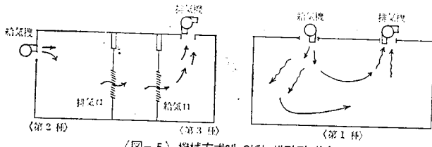
〈圖-5〉機械方式에 의한 새가지 換氣
