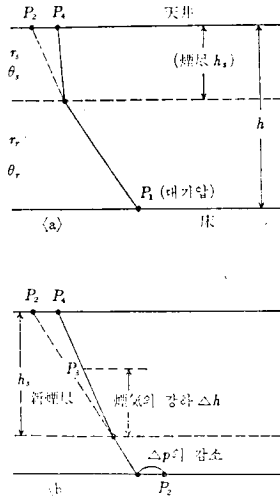
〈圖-4〉 廊下에 흐르는 煙氣의 安定, 不安定
