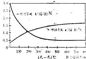
〈圖-3〉 煙氣의 두께와 속도
