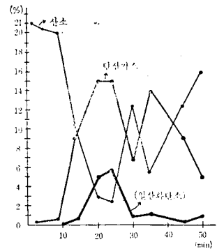
(圖-1) 火災室 空氣成分의 變化
