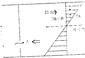
圖-7 開口部の 中性帶와 壓力
