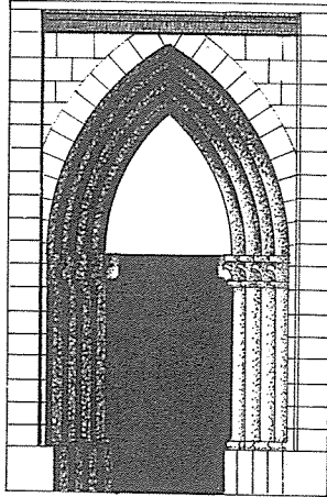
GOTHIC 고딕식
