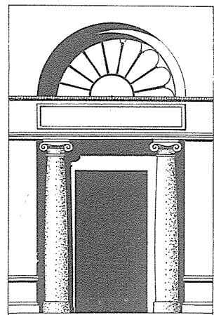
NEO-CLASSICAL 신·고전식
