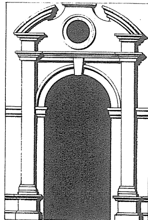
RENAISSANCE 르네상스식
