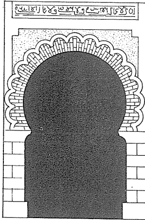
MOORISH 무어식
