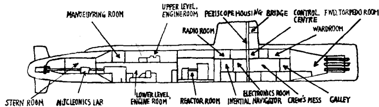
그림 6. 核潛水艦 Skate級의 內部概圖
