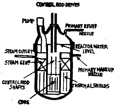
그림 17. CNSG 原子爐
