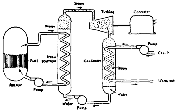
그림 3. 加壓水型原子爐
