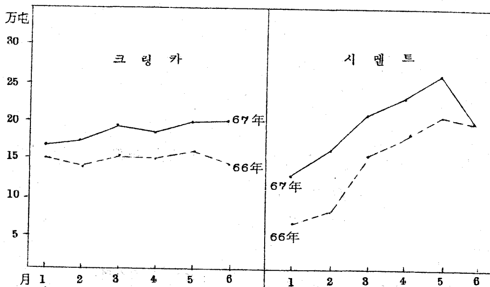
그림 1. 크렁카 및 시멘트生産趨勢
