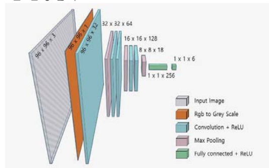
<그림 1> The Architecture of FashionNet
