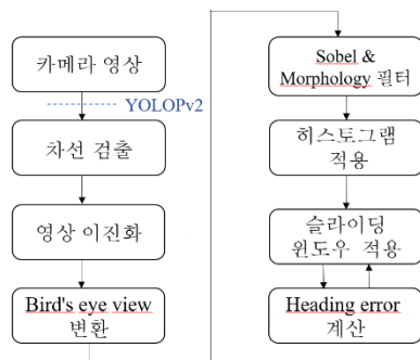
그림 1. 알고리즘 순서도
