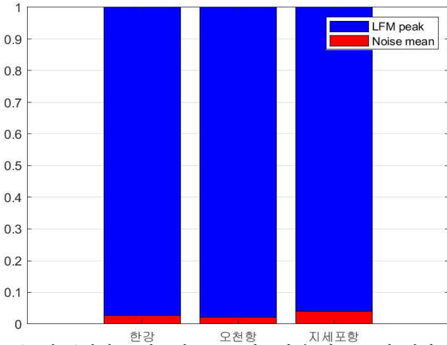
(그림 8) 실험 포인트별 LFM 상호상관 피크 크기 대비 잡음 평균
