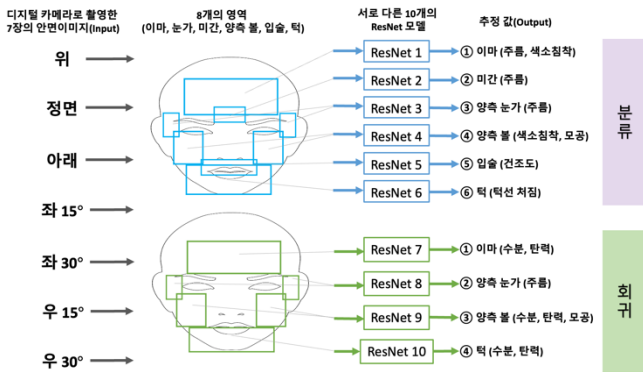
(그림 8) 7 장의 멀티뷰 이미지를 입력으로 받는 AI 모델개요
