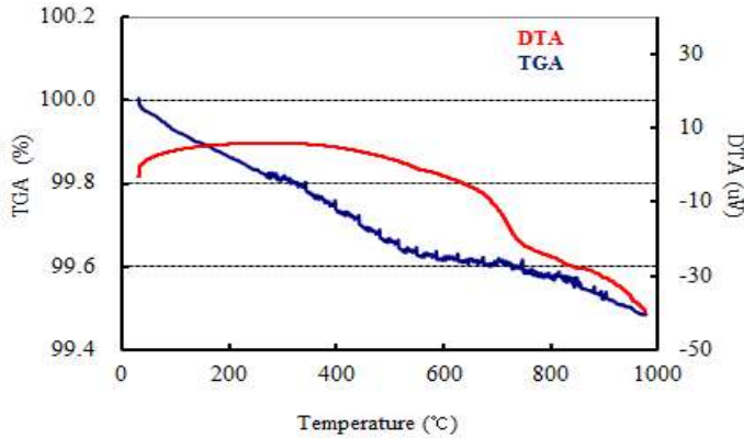
그림 2. 유리분말 TG-DTA
